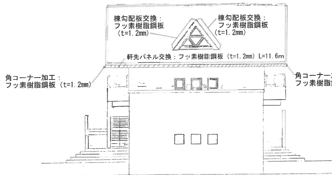
東立面図
