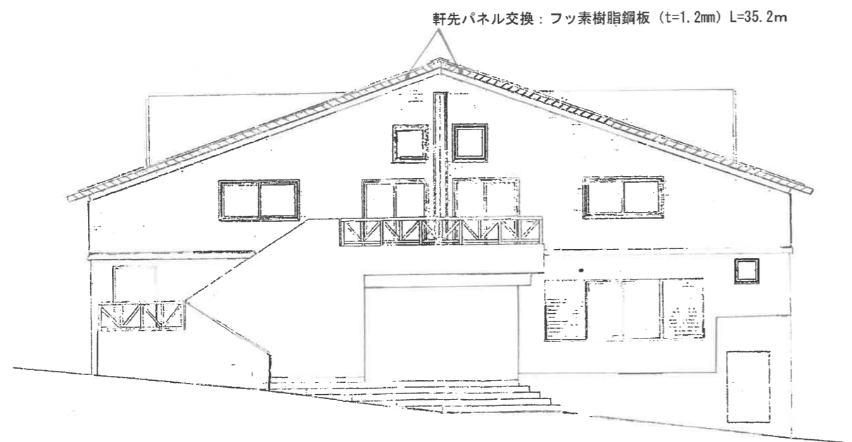
南立面図
