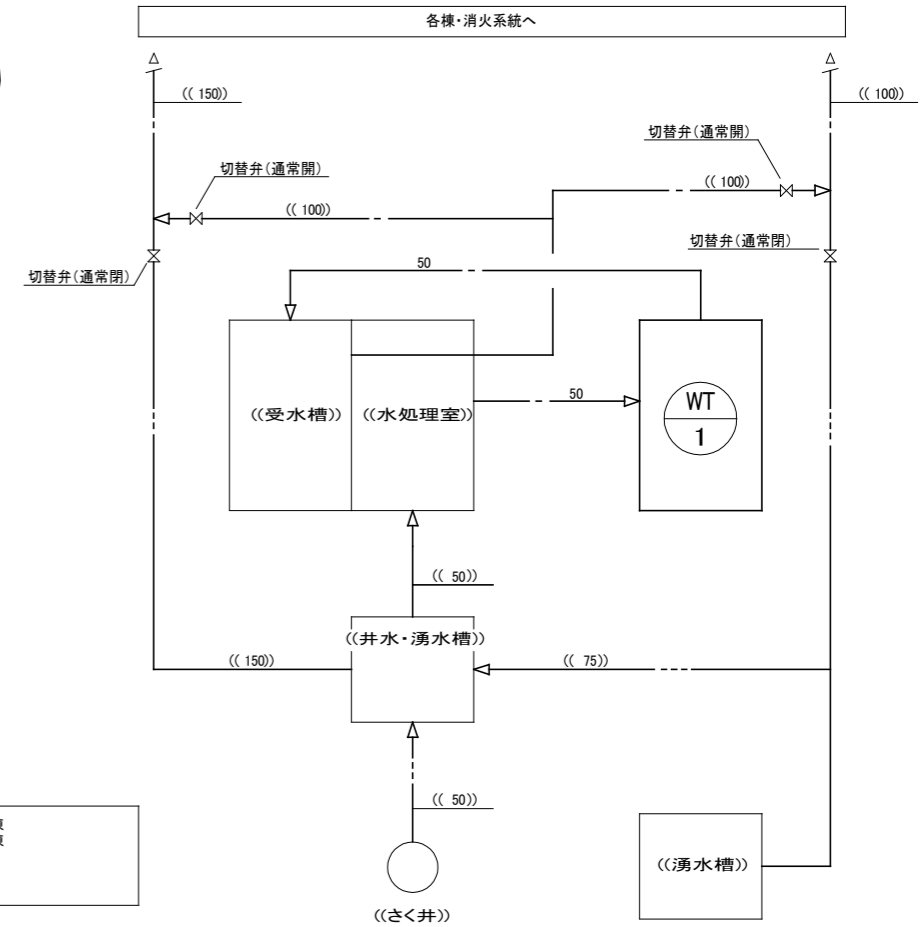
給水設備 フロー図 (改修後) S=N.S
