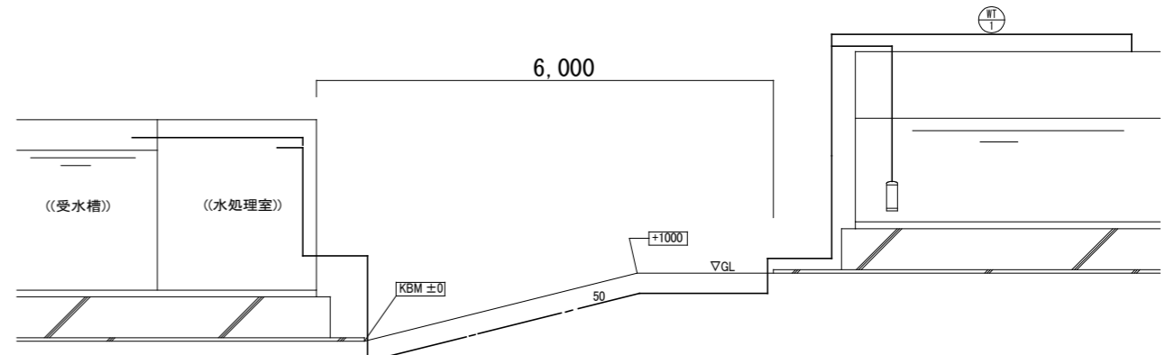
埋設配管要領図(浄水) N.S
