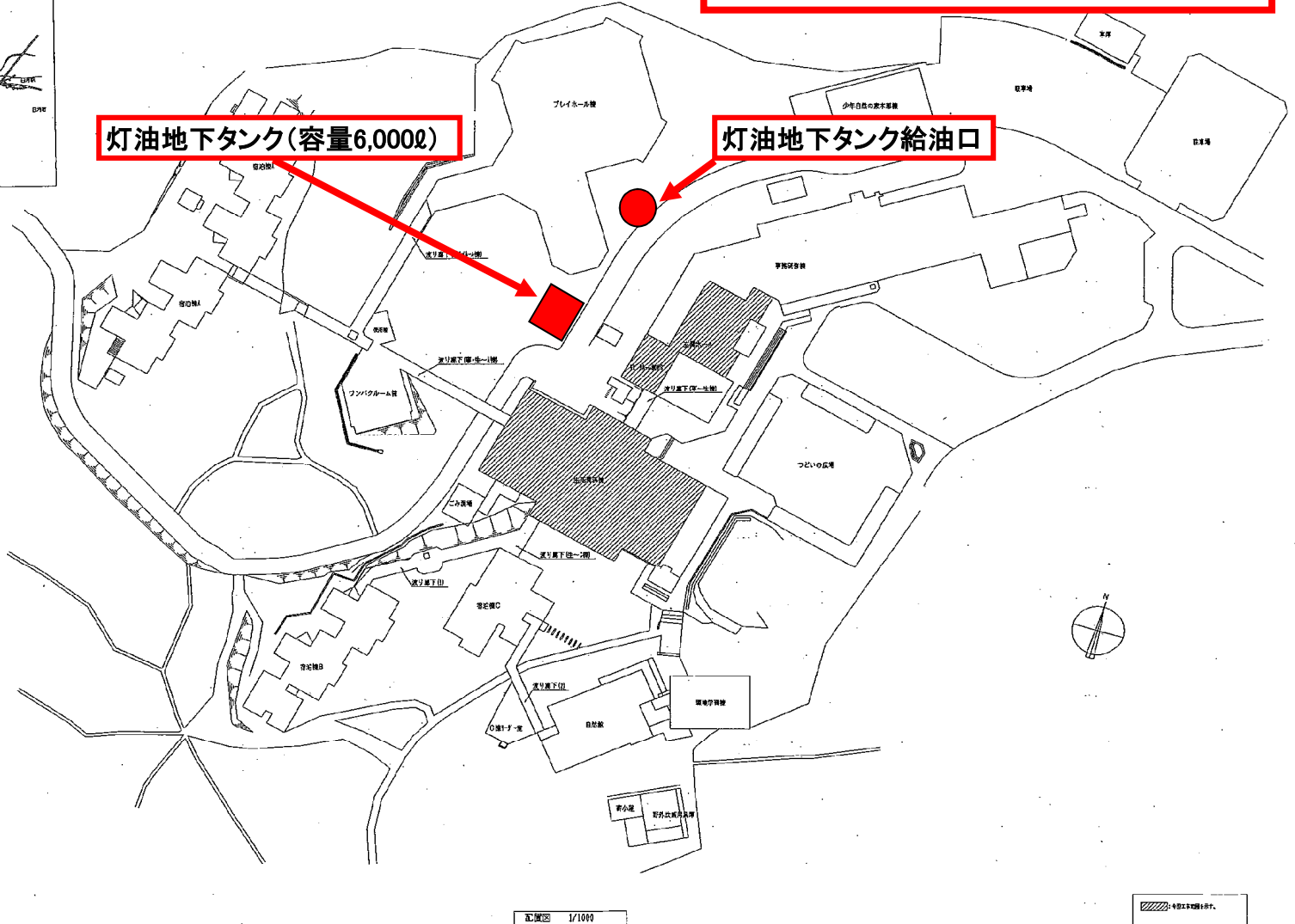
配置図 1/1000
