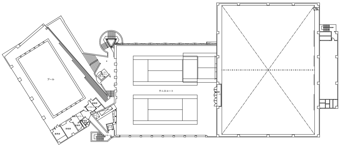
スポーツ棟 3階 平面図(1:400)
