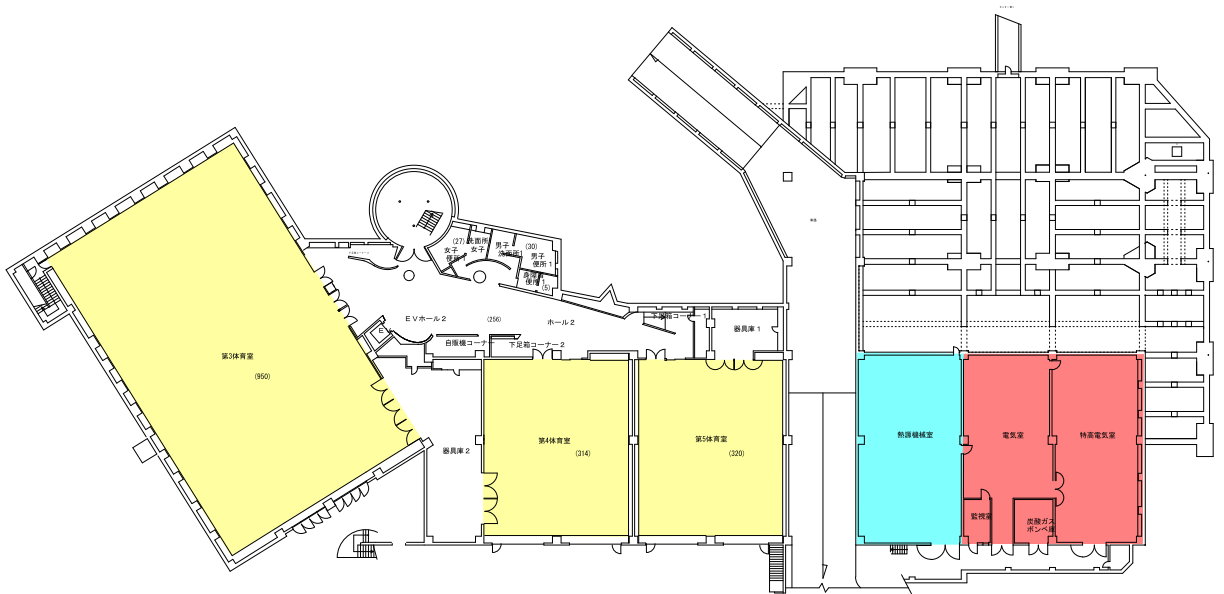
スポーツ棟 地下1・地下中1階 平面図(1:400)
